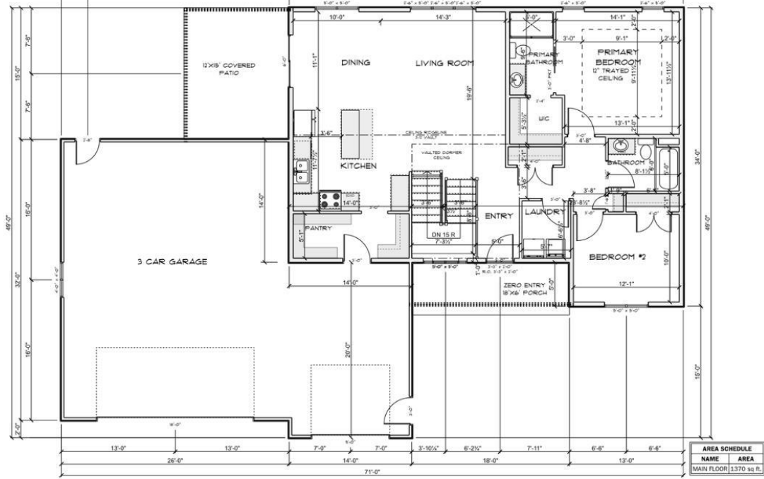
MAIN FLOOR SCALE: 1/8" = 1'-0"
